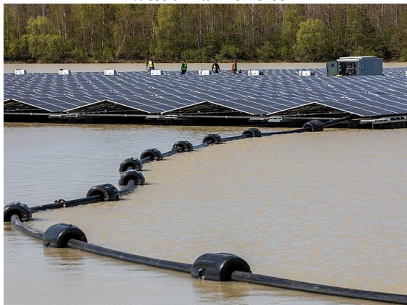
Rysunek 7 Pływająca farma fotowoltaiczna na zbiorniku Silberseen und Schmaloe Heide w Nadrenii Północnej Westfalii w Niemczech
